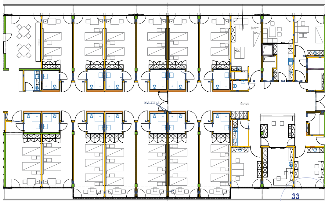
Neubau Frauenklinik: Ausschnitt aus dem Grundriss 1. Obergeschoss
